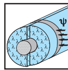
Wärmebrücke \psi [W/(m·K)]
